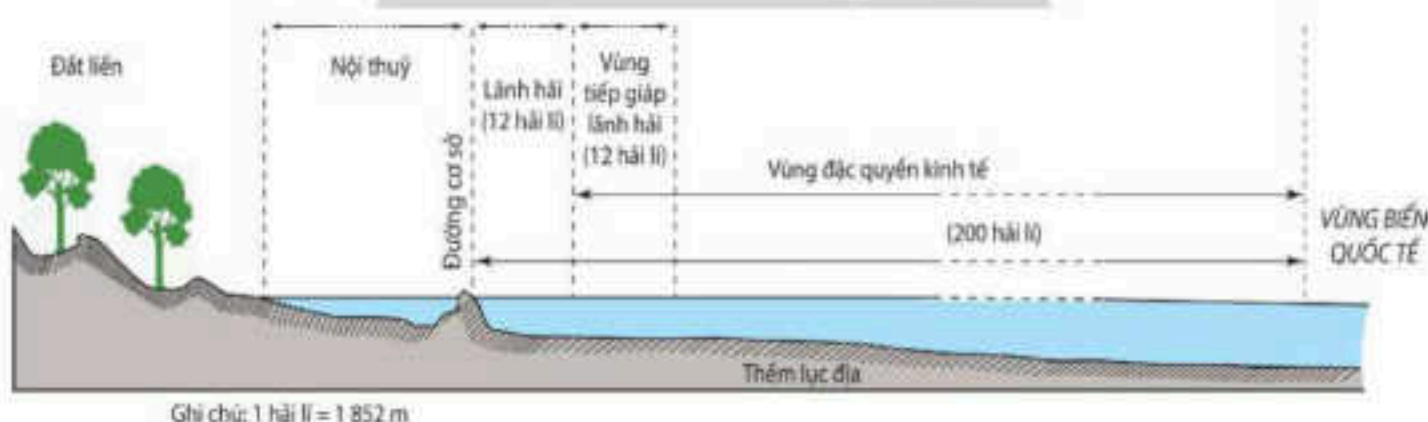
Hình 23.1. Sơ đồ mặt cắt khái quát các vùng biển Việt Nam (theo Luật Biển Việt Nam năm 2012)
