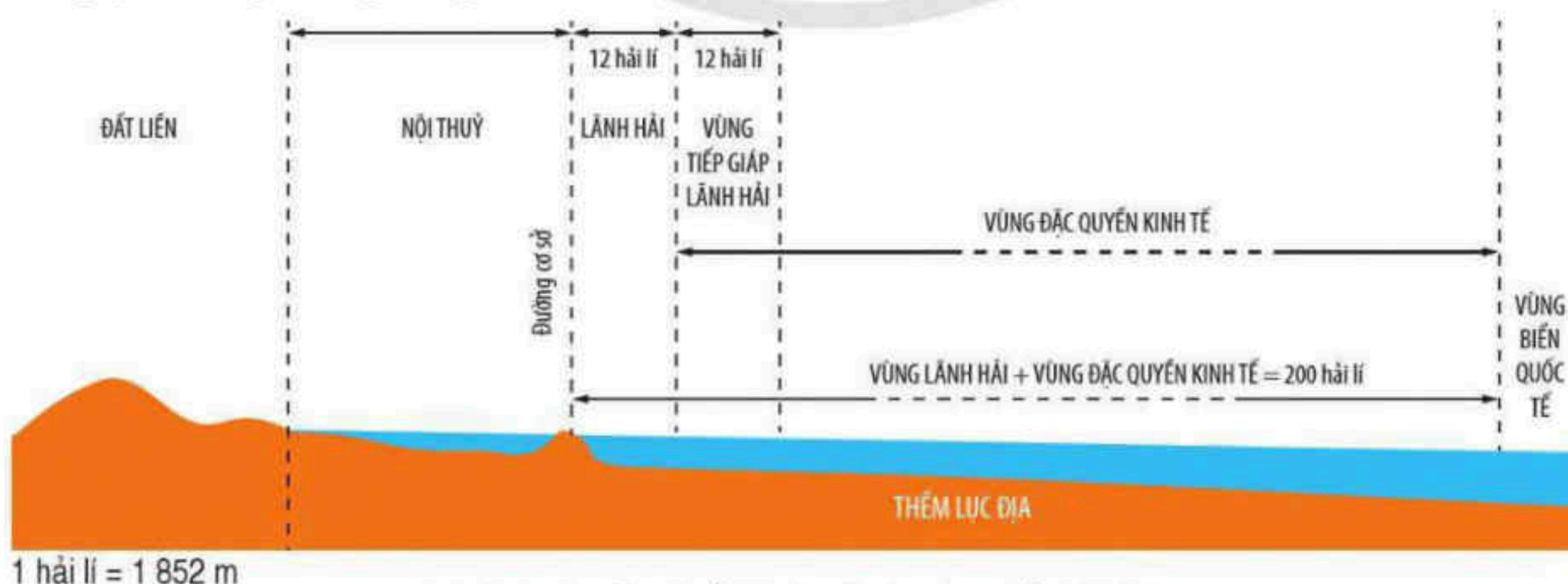
Hình 11.2. Sơ đồ mặt cắt khái quát các vùng biển Việt Nam
