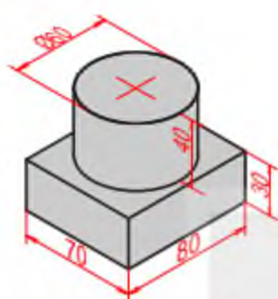
Hình 2.19. Gối đỡ
