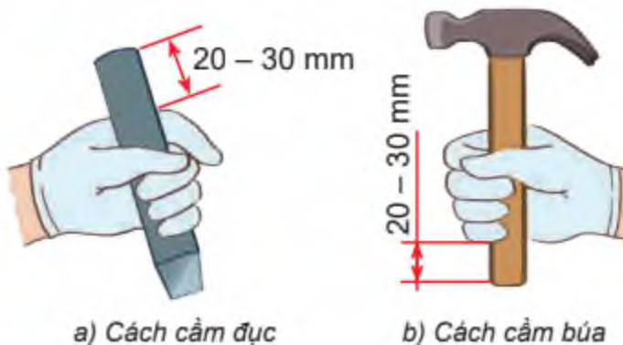
Hình 8.9. Cách cầm đục và búa
