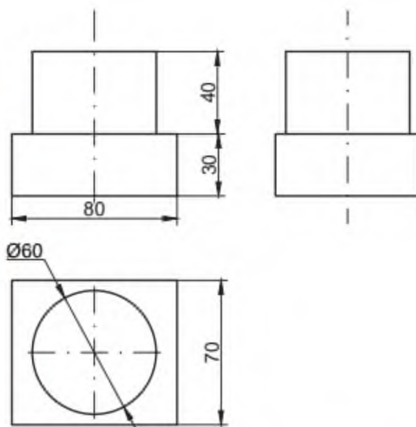
Hình 2.24. Tô nét, ghi kích thước
