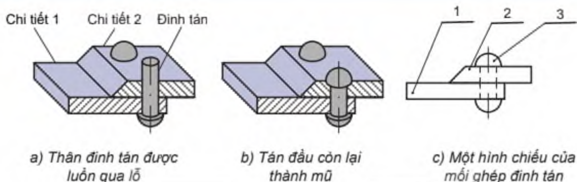
Hình 4.3. Mối ghép đỉnh tán
