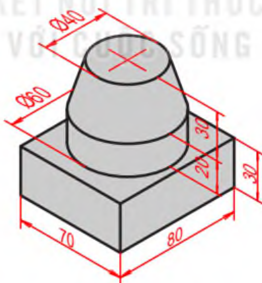
Hình 2.25. Giá đỡ
