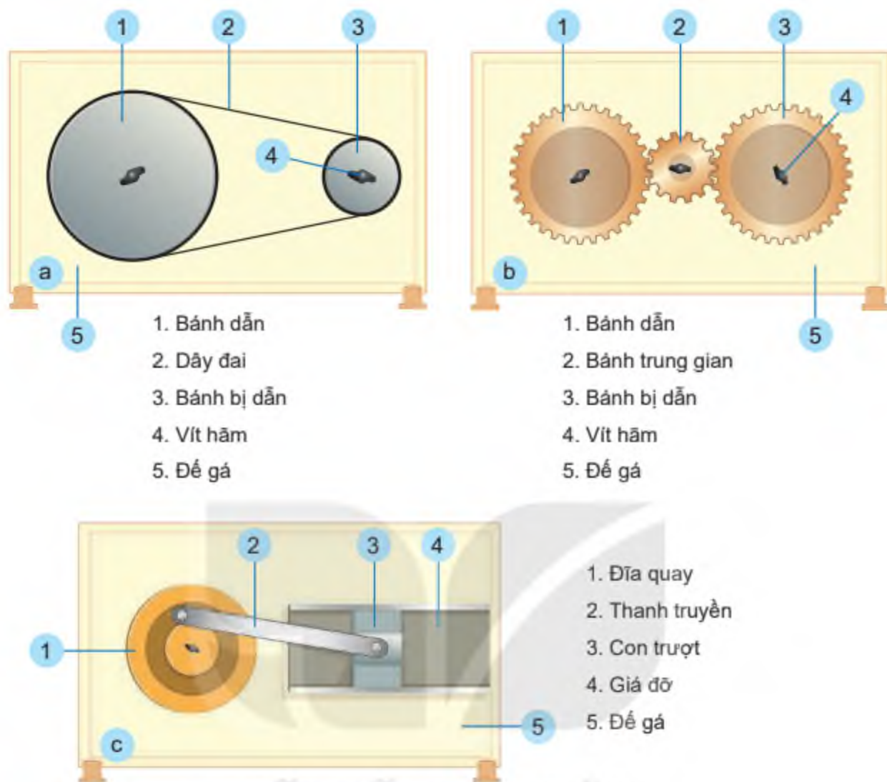
Hình 7.6. Bộ mô hình truyền và biến đổi chuyển động
