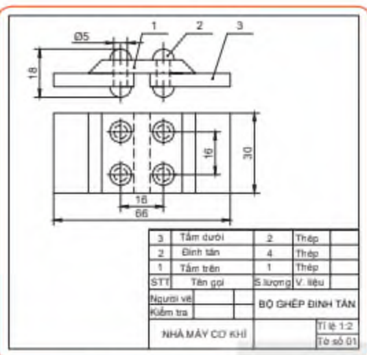
Hình 4.1. Bản vẽ lắp bộ ghép đinh tán
