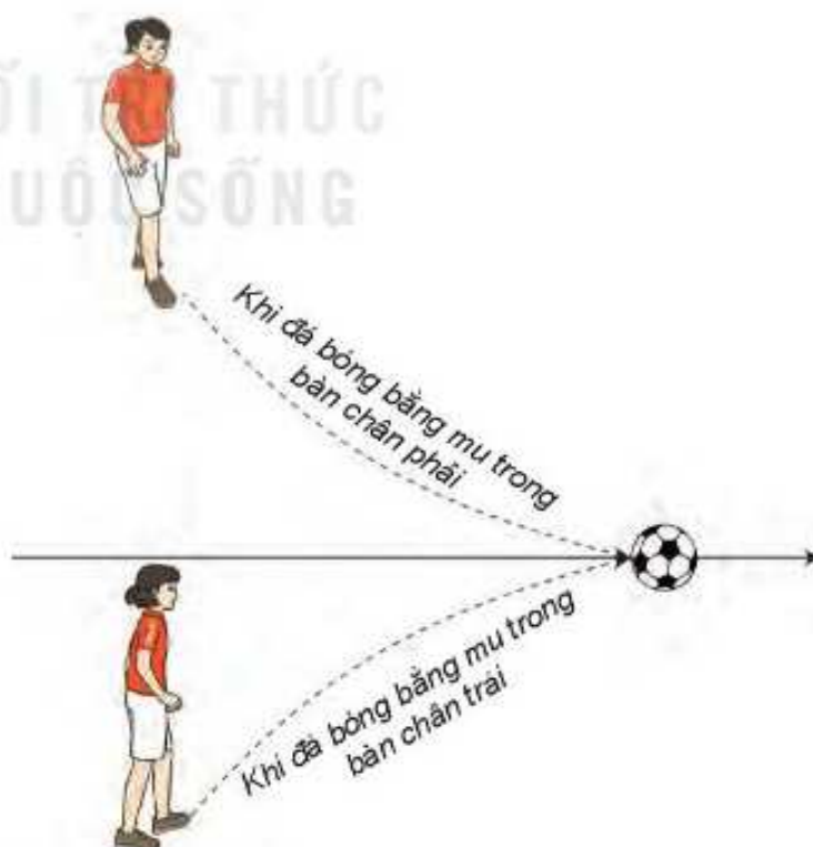
Hình 6. Hướng và vị trí xuất phát chạy đà
