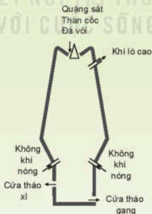
Hình 13.6 Sơ đồ lò cao sản xuất gang
