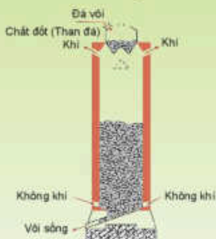
Hình 13.3 Sơ đồ lò nung vôi
