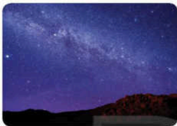
Ảnh chụp Ngân Hà từ Trái Đất
