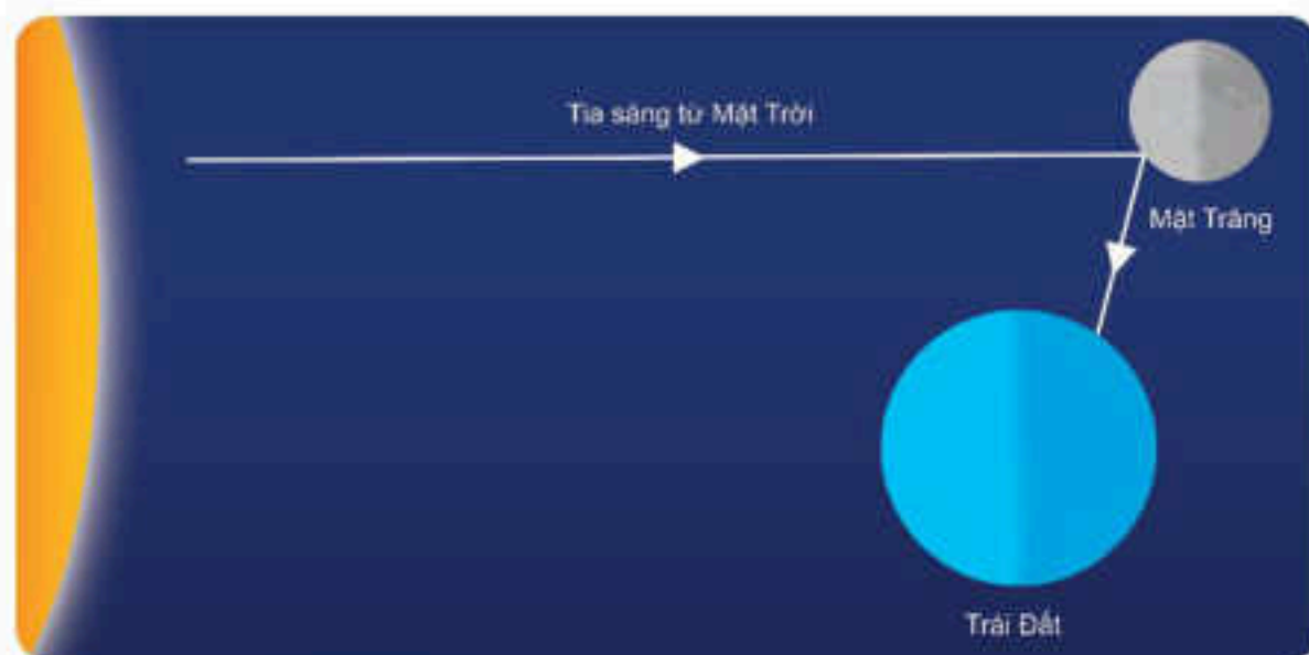
Hình 53.1 Mặt Trời – Mặt Trăng – Trái Đất
