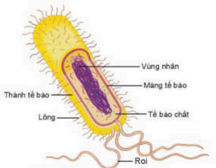
Hình 27.2 Cấu tạo một vi khuẩn
