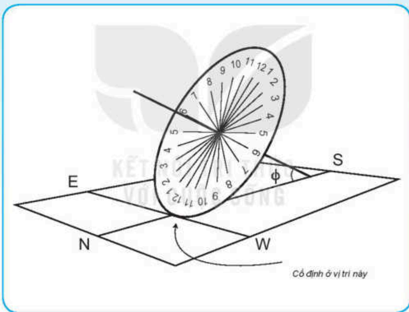
Hình 52.6 Cấu tạo của đồng hồ mặt trời
