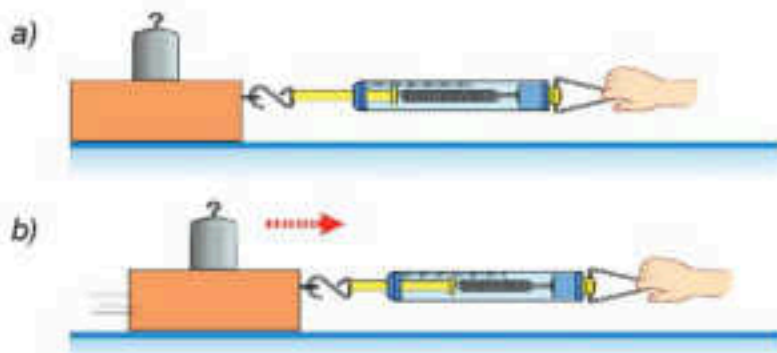
Hình 44.4 Thí nghiệm về các lực ma sát
