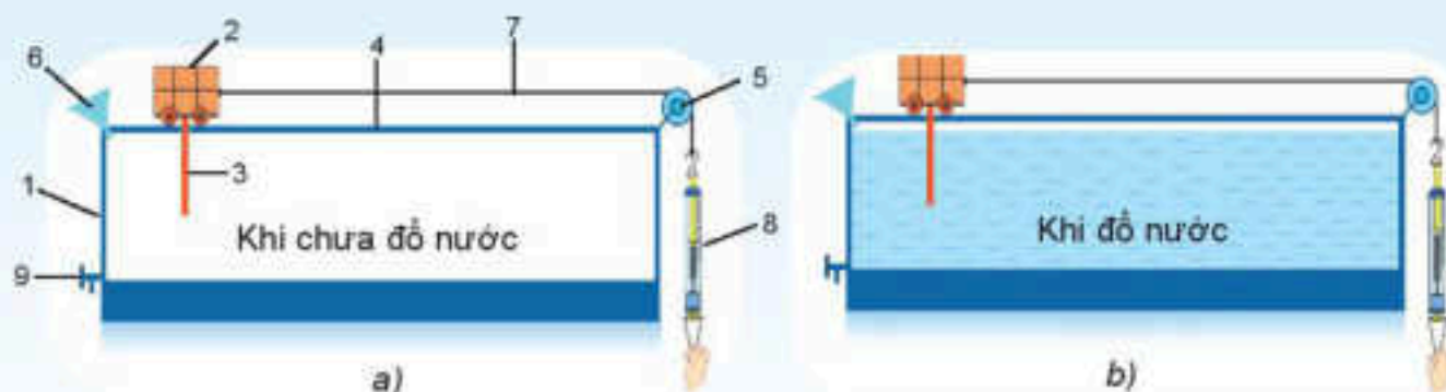
Hình 45.1 Thí nghiệm về lực cản
