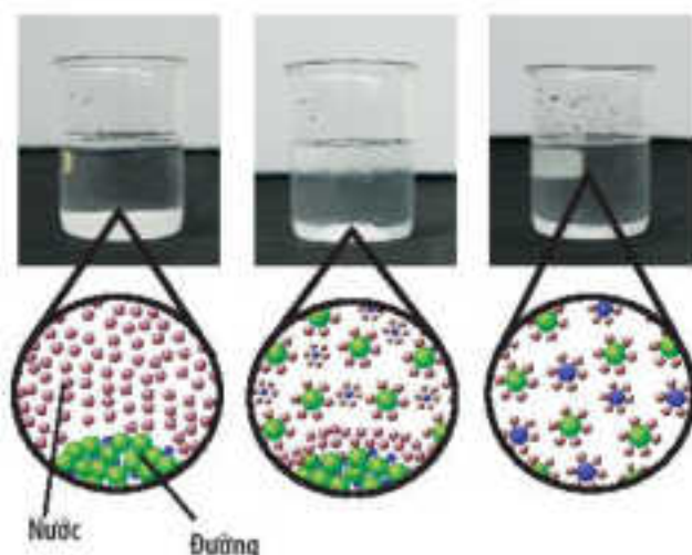
▲ Hình 15.8. Quá trình tạo dung dịch đường
