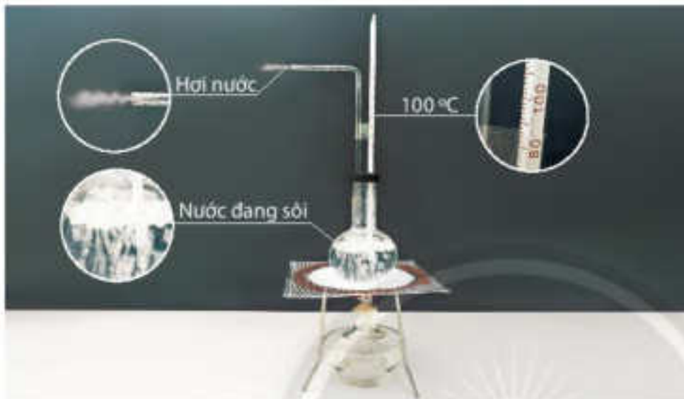
▲ Hình 8.7. Đo nhiệt độ sôi của nước
