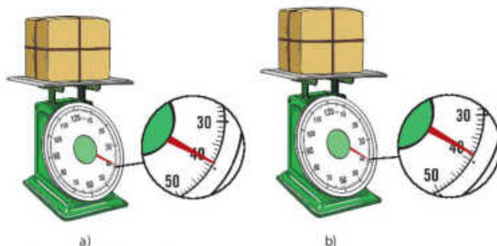
▲ Hình 5.6. Đọc kết quả đo khối lượng
