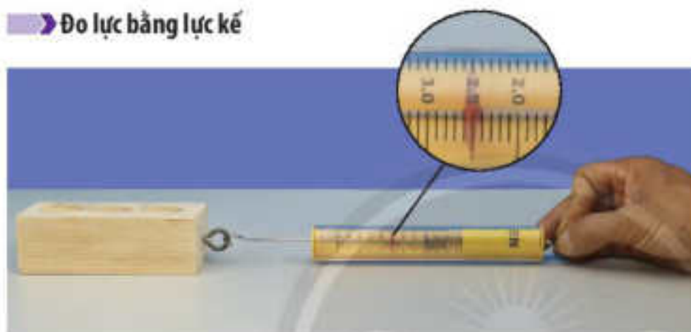
▲ Hình 39.3. Đo lực bằng lực kế
