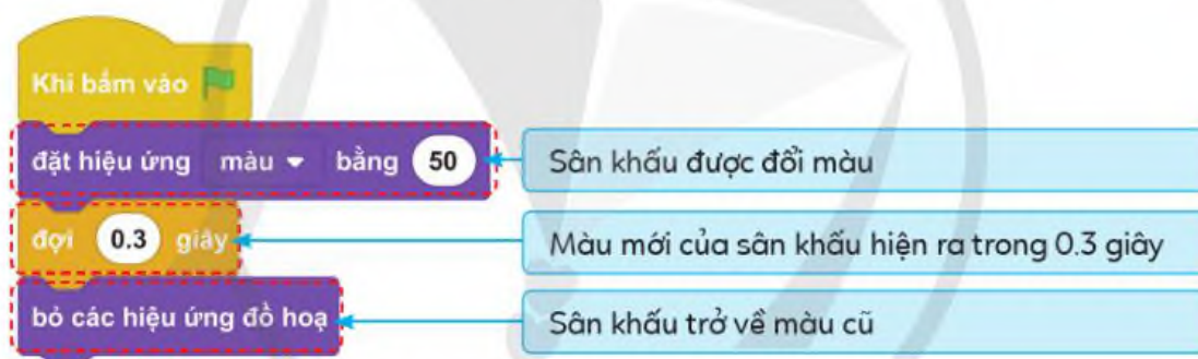
Hình 5. Chương trình cho phong nền sân khấu
