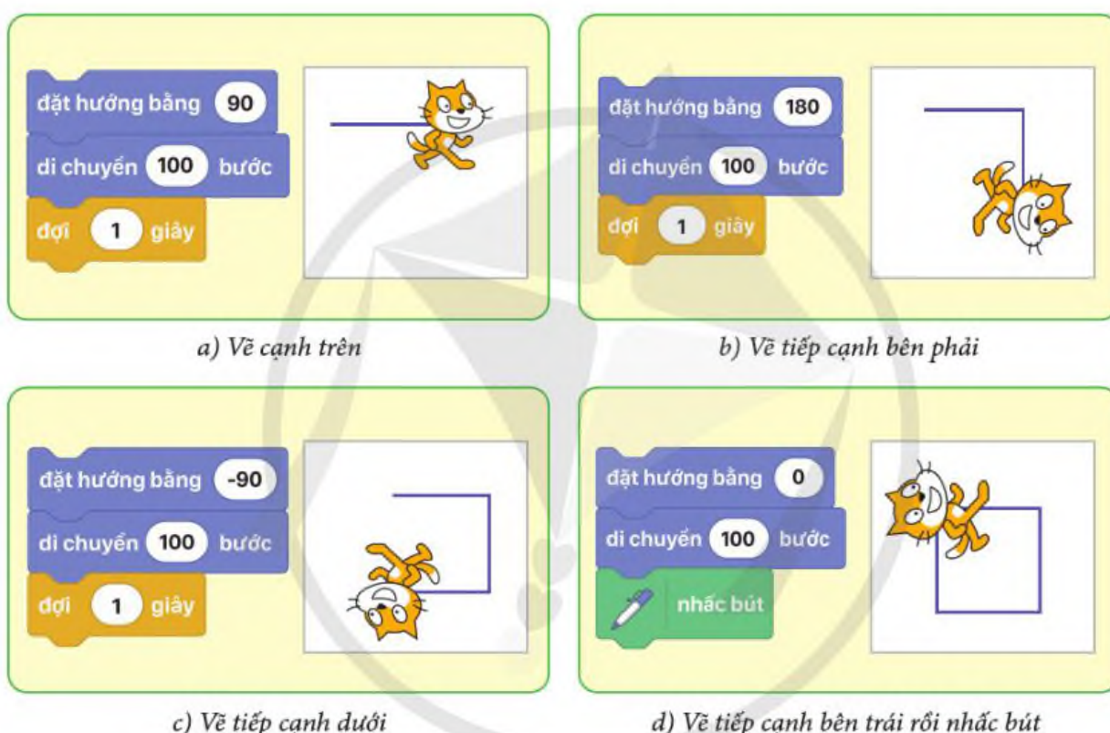
Hình 3. Các khối lệnh vẽ từng cạnh của hình vuông và kết quả thực hiện vẽ
