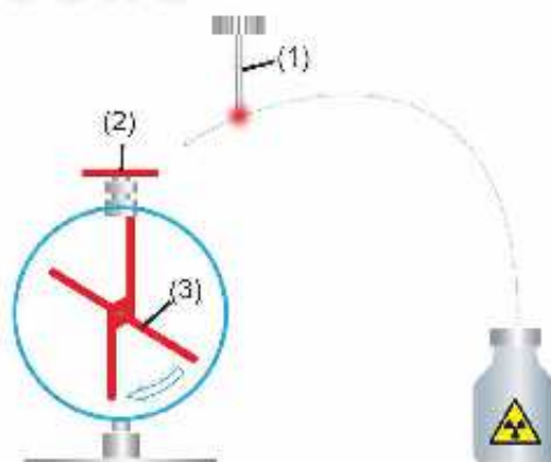
Hình 25.1. Thí nghiệm đưa mẫu phóng xạ lại gần tĩnh điện kế
