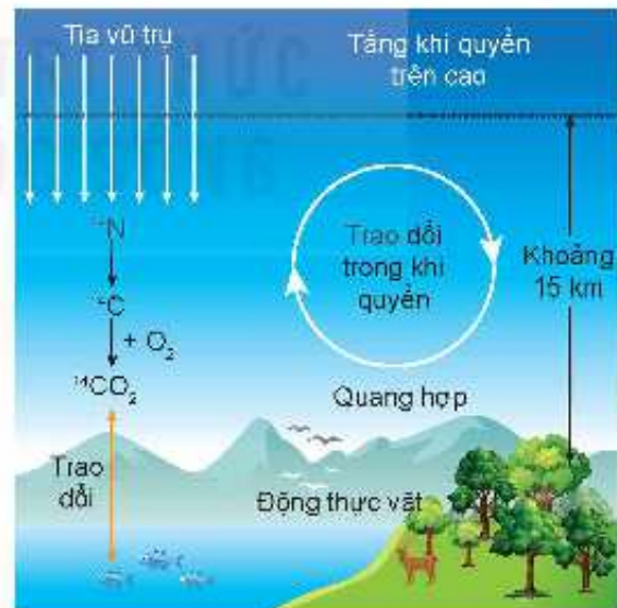
Hình 23.6. Quy trình hình thành ^{14}_6C trên Trái Đất
