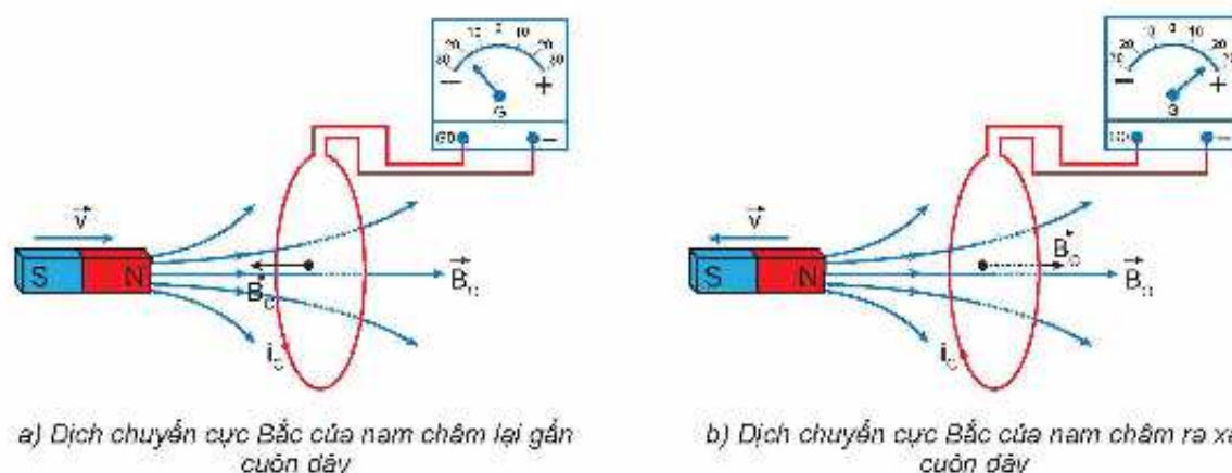
Hình 16.8. Thí nghiệm về chiều dòng điện cảm ứng. \vec{B}_n là kí hiệu cảm ứng từ của từ trường do dòng điện cảm ứng i_c trong cuộn dây sinh ra; \vec{B}_n là cảm ứng từ của từ trường nam châm
