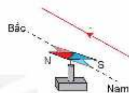
Hình 14.2. Thí nghiệm của Oersted (Ơ-xtét) về tương tác giữa dòng điện và kim nam châm
