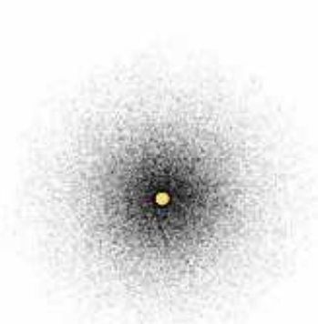
b) Mô hình đám mây electron
