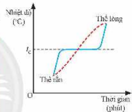
▲ Hình 1.12. Đồ thị phản ánh sự thay đổi nhiệt độ theo thời gian trong quá trình chuyển thể từ rắn sang lỏng của chất rắn kết tinh (đường liên tục màu xanh) và của chất rắn vô định hình (đường nét đứt màu đỏ)
