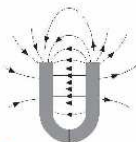
▲ Hình 9P.2. Đường sức từ xung quanh nam châm chữ U
