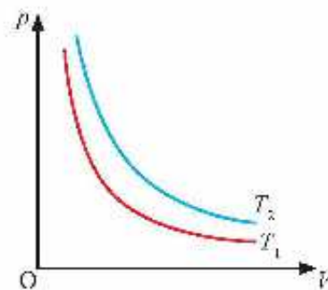
▲ Hình 6.4. Các đường đẳng nhiệt của một khối khí tương ứng với các nhiệt độ T_1 và T_2 ( T_1 < T_2 )
