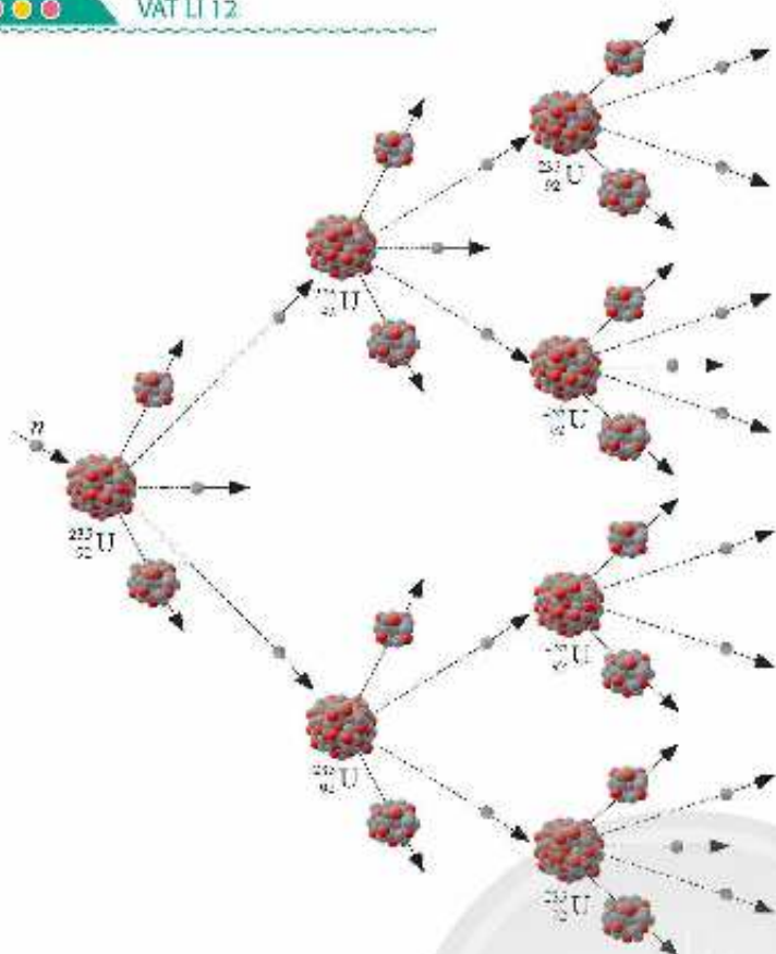
▲ Hình 16.3. Sơ đồ minh họa phản ứng dây chuyền với ^{235}\text{U}
