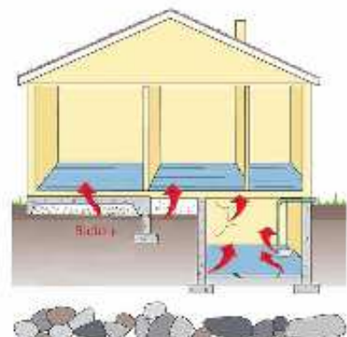
▲ Hình 18.2. Khí radon ( {}^{222}_{86}\text{Rn} ) thâm nhập vào nhà từ lòng đất (các mũi tên chỉ đường thâm nhập của chất khí này)
