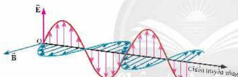
▲ Hình 12.8. Mô hình sự lan truyền sóng điện từ
