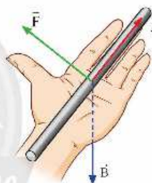
▲ Hình 10.4. Quy tắc bàn tay trái để xác định chiều của lực từ
