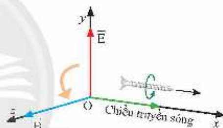
▲ Hình 12.9. Minh họa quy tắc vận định ốc
