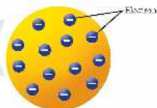
▲ Hình 14.1. Mô hình nguyên tử của Thompson
