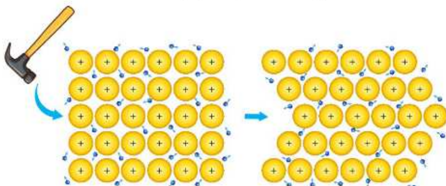
Hình 13.3. Minh hoạ quá trình trượt của các cation kim loại khi bị tác động bởi lực
