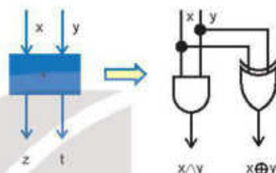
Hình 4.10. Mạch logic thực hiện phép cộng
