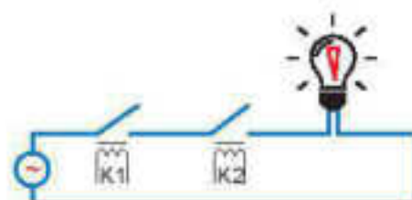
Hình 4.4. Mạch điện thực hiện phép nhân logic
