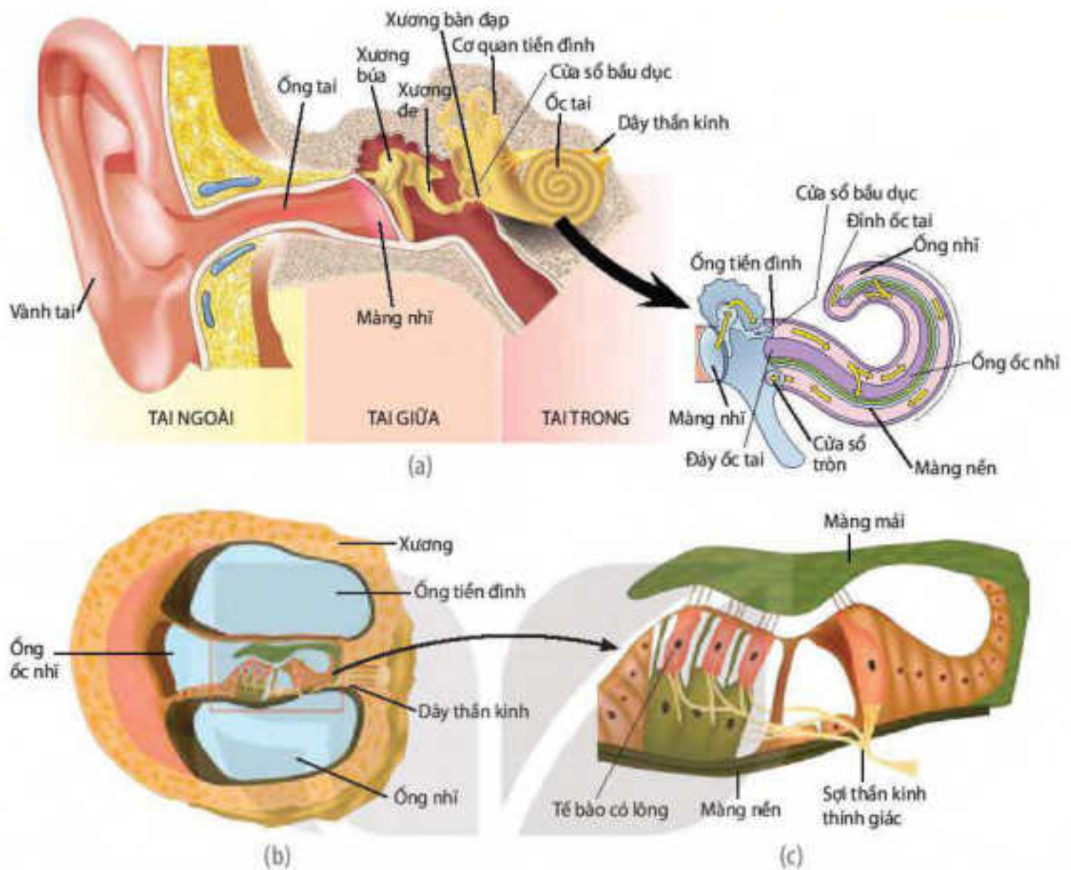
Hình 17.14. Tai giữa và ốc tai được vẽ dài ra (a), tiết diện cắt ngang ốc tai (b), Các tế bào có lông và màng mái trên màng nền (c)
