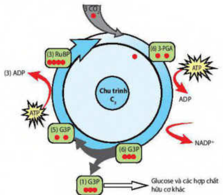
Hình 4.3. Chu trình \text{C}_3
