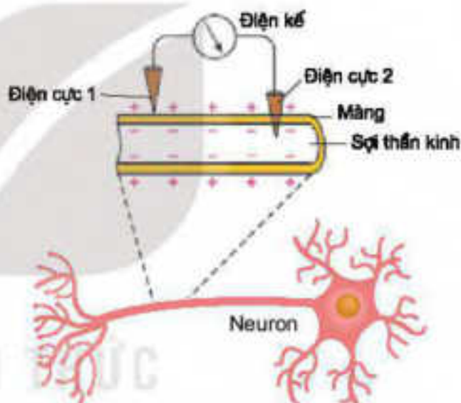
Hình 17.5. Sơ đồ đo điện thế nghỉ
