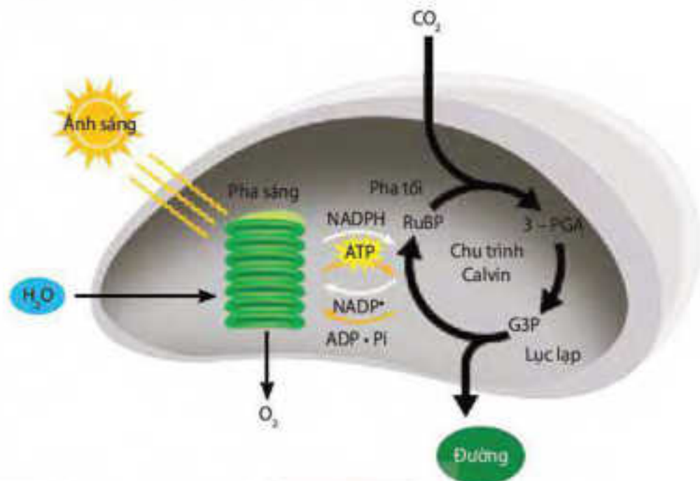
Hình 4.2. Hai pha của quá trình quang hợp
