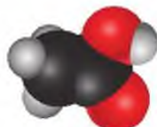
b) Mô hình đặc
