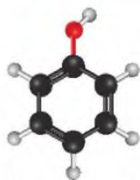
a) Mô hình quả cầu – thanh nối
