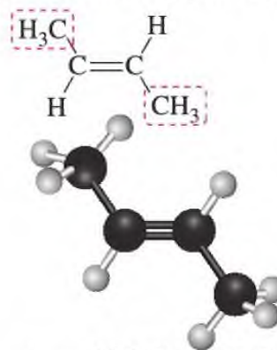
Hình 13.3. Công thức cấu tạo và mô hình phân tử của cis -but-2-ene (a) và trans -but-2-ene (b)
