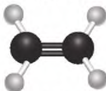
Hình 13.1. Mô hình phân tử ethene
