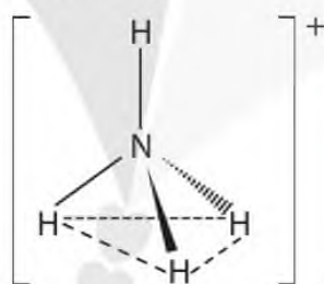
Hình 5.2. Dạng hình học của ion ammonium
