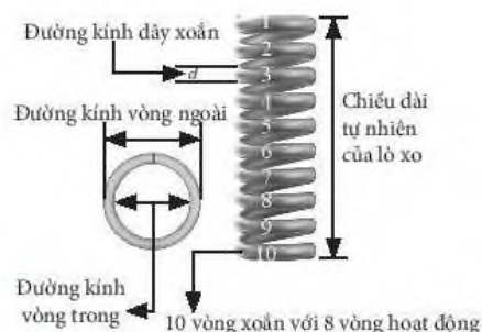
▲ Hình 23.7. Các yếu tố ảnh hưởng đến độ cứng của một lò xo
