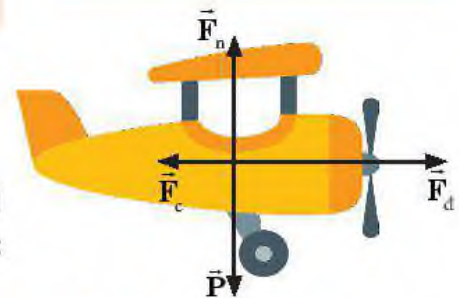
Hình 10.9. Minh họa trường hợp vật chịu nhiều lực đồng thời tác dụng
