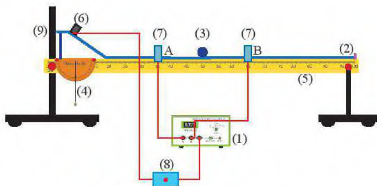
Hình 6.2. Bố trí thí nghiệm đo tốc độ
