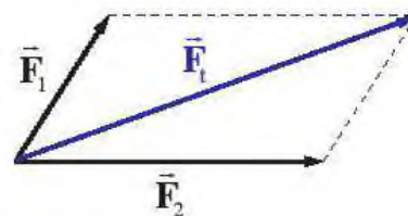
▲ Hình 13.3. Minh họa cách tổng hợp lực bằng quy tắc hình bình hành
