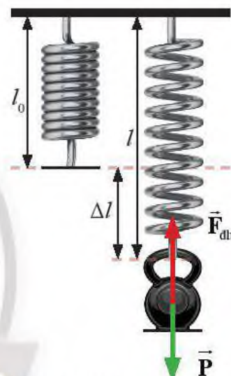
Hình 23.3. Lò xo bị dãn khi treo vật vào
