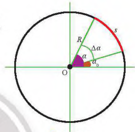
Hình 20.7. Độ dịch chuyển góc \Delta\alpha
