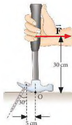
Hình 14P.2. Nhổ đinh bằng búa
