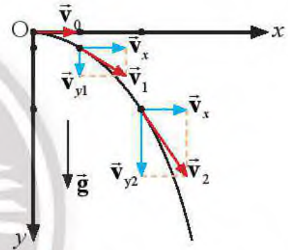
Hình 9.4. Biểu diễn vận tốc của vật và hình chiếu của nó lên hai trục Ox , Oy trong quá trình chuyển động
