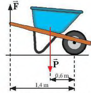
▲ Hình 14.11. Xe đẩy vật liệu
