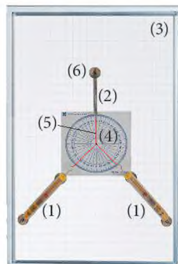
▲ Hình 13.11. Gợi ý bố trí thí nghiệm
