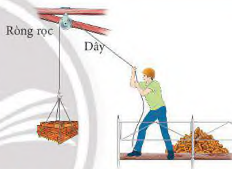
▲ Hình 11.13. Kéo gạch bằng ròng rọc
