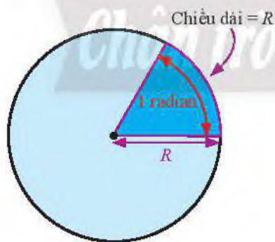
▲ Hình 20.3. Minh họa góc có số đo 1 rad
