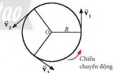
▲ Hình 20.11. Vận tốc trong chuyển động tròn đều
