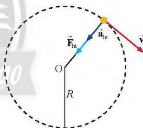
▲ Hình 21.2. Gia tốc hướng tâm và lực hướng tâm trong chuyển động tròn đều
