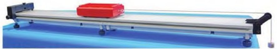
Hình 1.2. Thí nghiệm khảo sát liên hệ giữa lực và gia tốc
