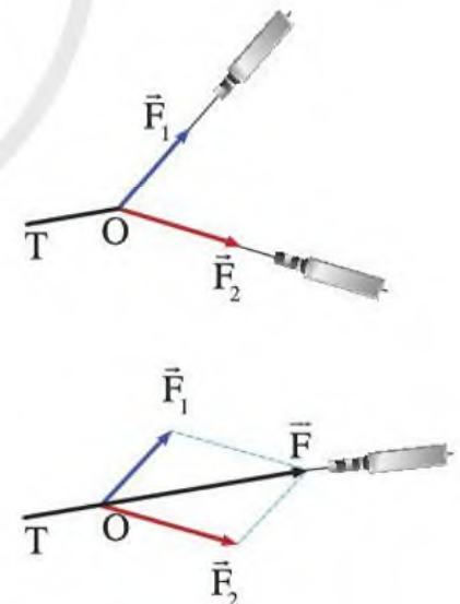
Hình 5.2. Lực F gây ra tác dụng lên dây cao su OT giống hệt khi F_1 và F_2 tác dụng đồng thời lên dây.
