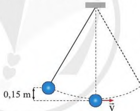
Hình 2.5. Chuyển động của con lắc
