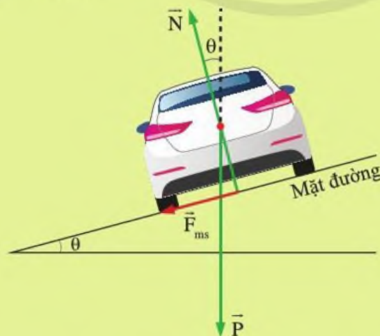
Hình 1.10. Ô tô chuyển động trên mặt đường nghiêng
