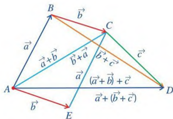
Hình 53. Minh họa tính chất phép cộng các vectơ
