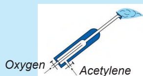
Hình 15.1. Sơ đồ cấu tạo đèn xì oxygen-acetylene
