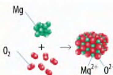
▲ Hình 12.1. Magnesium phản ứng với oxygen
