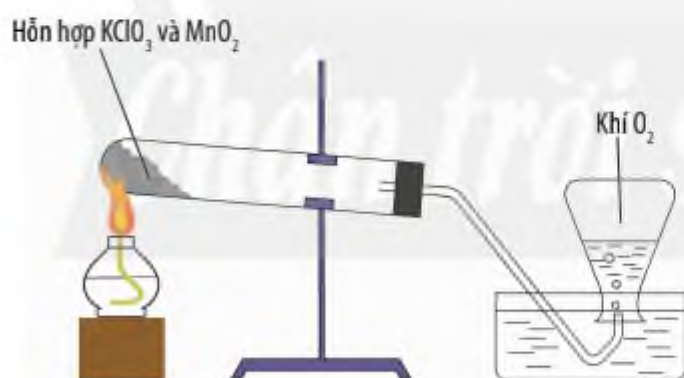
▲ Hình 13.4. Nhiệt phân potassium chlorate
