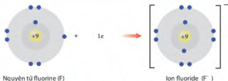
Hình 8.4. Sự hình thành ion F^-
