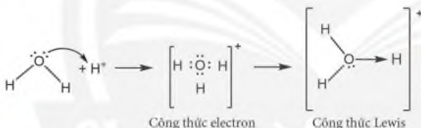
▲ Hình 10.4. Sơ đồ tạo liên kết cho nhận trong ion hydronium H_3O^+
