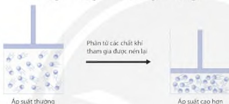
Hình 16.5. Minh hoạ khi tăng áp suất của các chất khí tham gia phản ứng
