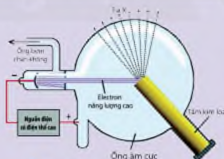
▲ Mô hình thí nghiệm khảo sát bản chất tự nhiên của tia X của Henry Moseley
