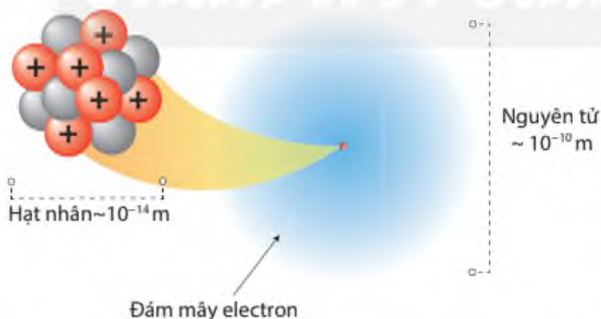
▲ Hình 2.6. Đường kính nguyên tử, hạt nhân trong nguyên tử carbon
