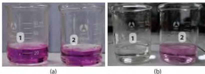
▲ Hình 16.3. Thí nghiệm ảnh hưởng của nhiệt độ đến tốc độ phản ứng
