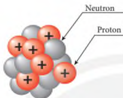
▲ Hình 2.5. Thành phần hạt nhân nguyên tử
