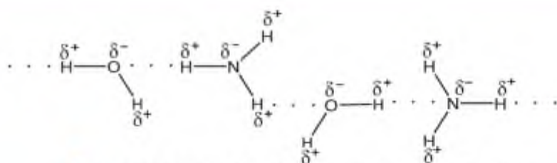
▲ Hình 11.5. Liên kết hydrogen giữa ammonia và nước
