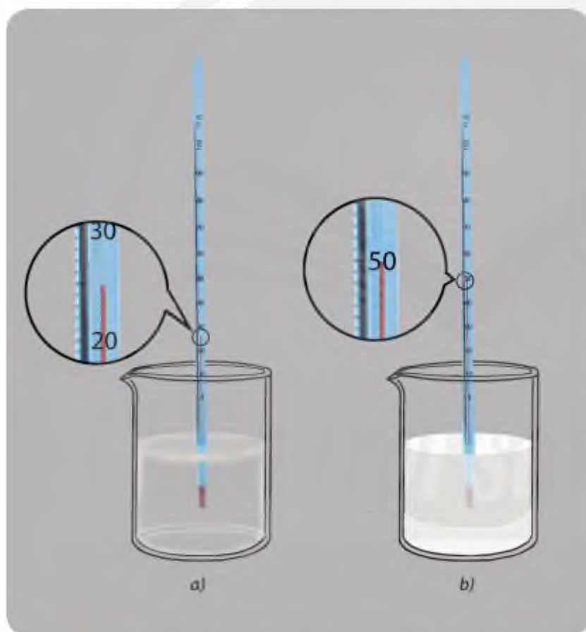
▲ Hình 13.2. Minh hoạ vôi sống phản ứng với nước
