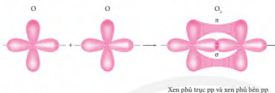
▲ Hình 10.8. Sự xen phủ các AO hình thành liên kết \sigma và liên kết \pi trong phân tử oxygen
