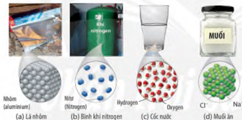
▲ Hình 1.1. Một số đơn chất và hợp chất
