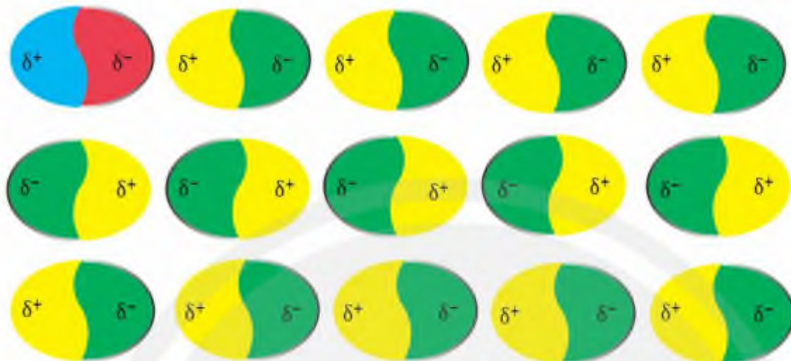
▲ Hình 11.8. Mạng lưới tương tác lưỡng cực cảm ứng được tạo thành bởi lưỡng cực tạm thời
