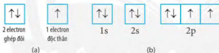
▲ Hình 4.9. (a) Electron ghép đôi và electron độc thân; (b) Sự sắp xếp electron trên các orbital của nguyên tử oxygen
