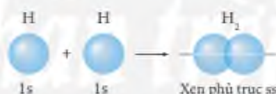
▲ Hình 10.5. Sự xen phủ giữa hai orbital 1s của hai nguyên tử hydrogen hình thành liên kết \sigma trong phân tử hydrogen
