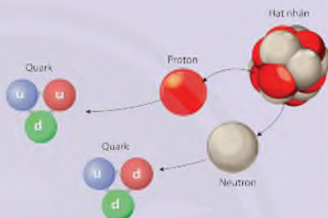
▲ Cấu tạo của proton và neutron
