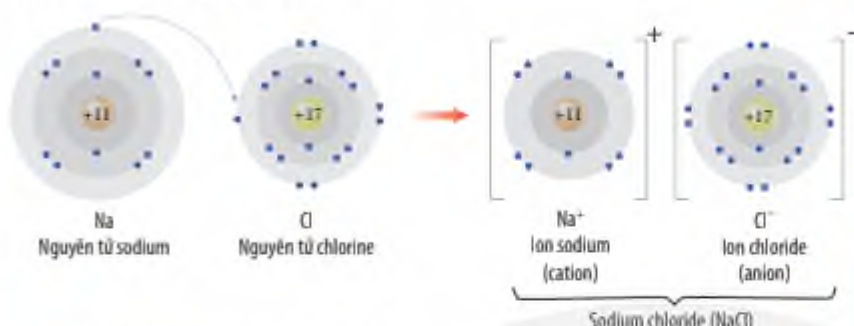
▲ Hình 9.2. Minh hoạ sự hình thành liên kết ion trong phân tử NaCl
