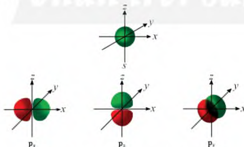
▲ Hình 4.4. Hình dạng của các orbital s và p
