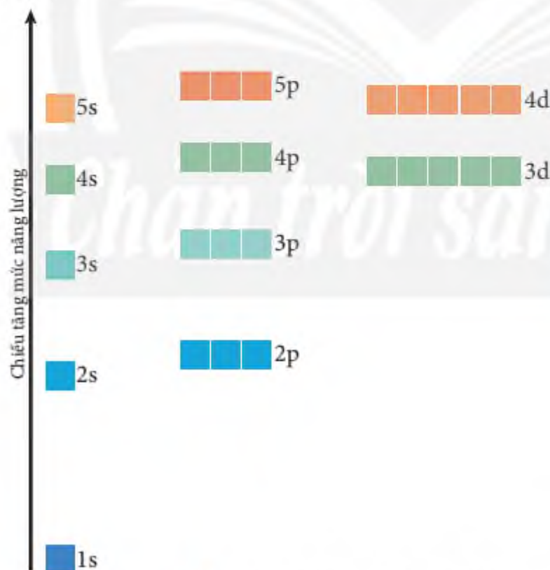
▲ Hình 4.7. Mối quan hệ về mức năng lượng của các orbital trong những phân lớp khác nhau
