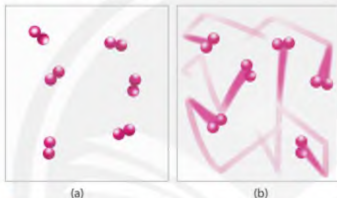
▲ Hình 16.4. Hình minh họa chuyển động của chất phản ứng khi chưa đun nóng (a) và được đun nóng (b)
